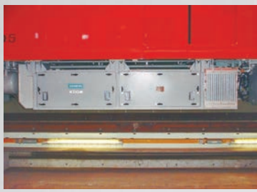
“歌う電車”の正体、シーメンス社製のVVVFインバーター装置。VVVFはVariable Voltage Variable Frequency (可変電圧可変周波数)の頭文字。
